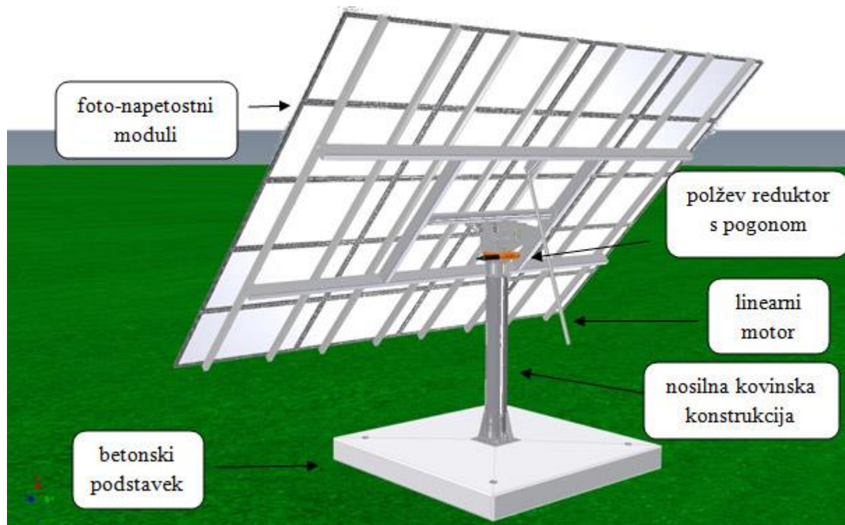
Slika 5: Dvoosni sledilnik sonca, ki omogoča optimalno sledenje soncu (vir: spletna stran Vrata Deržič)
