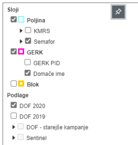
Slika 7: Seznam slojev
